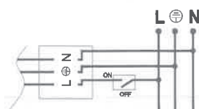
A. Standard function
